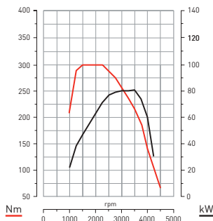
DCI 2.3 - 110 CV VERSIÓN COMBI-BUS 9 PLAZAS (EURO 6)
