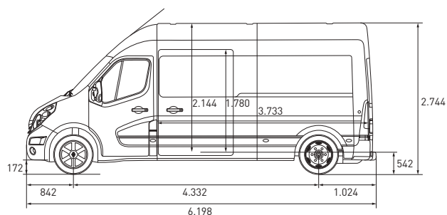
E20 VOLADIZO TRASERO CORTO H3 PROPULSIÓN
