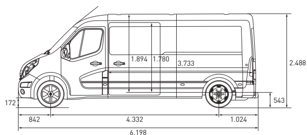
E20 VOLADIZO TRASERO CORTO H2 PROPULSIÓN
