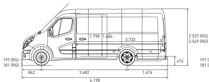
E30 VOLADIZO TRASERO LARGO H2
